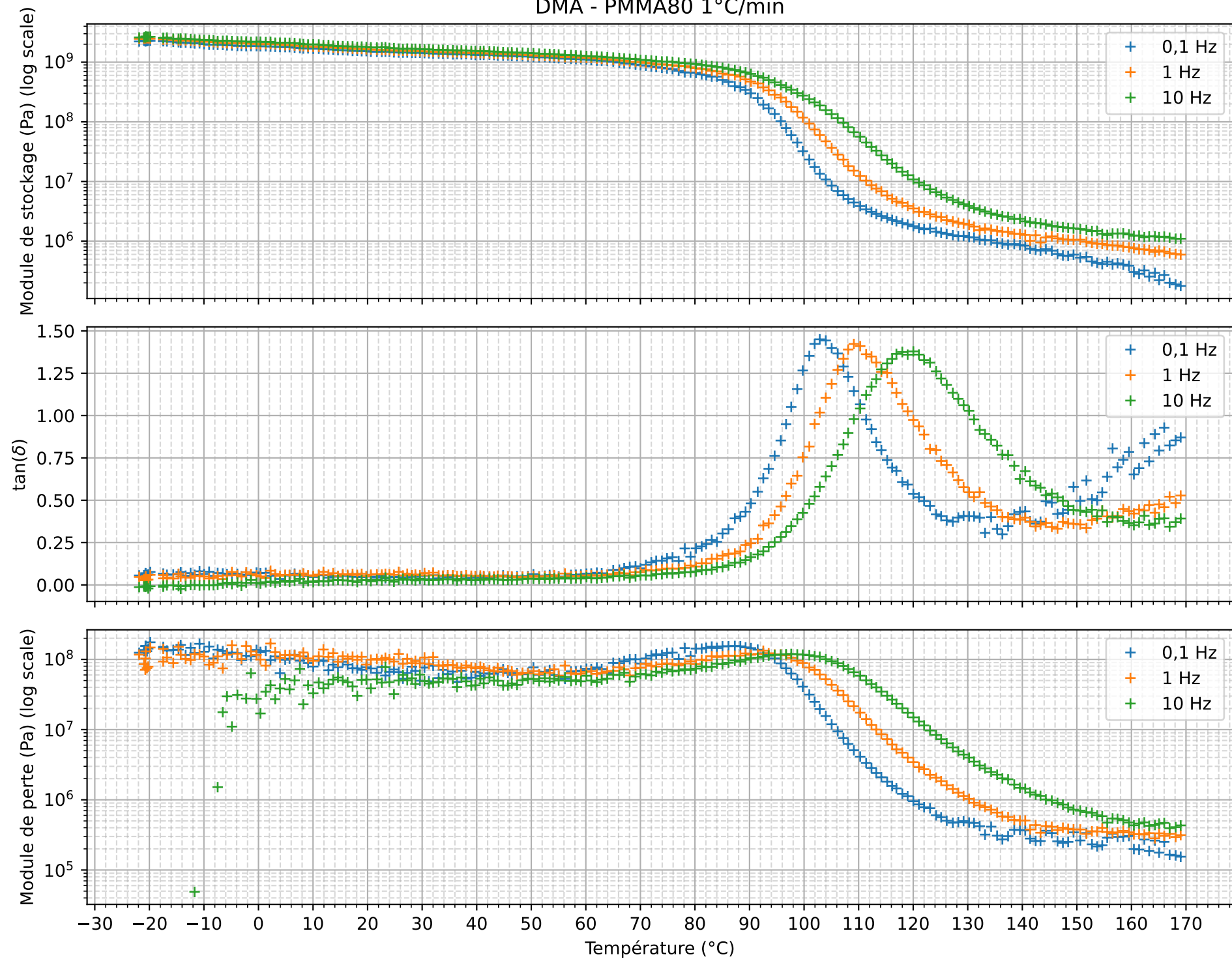
DMA - PMMA80 1°C/min
